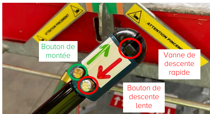
Poignée de commande
