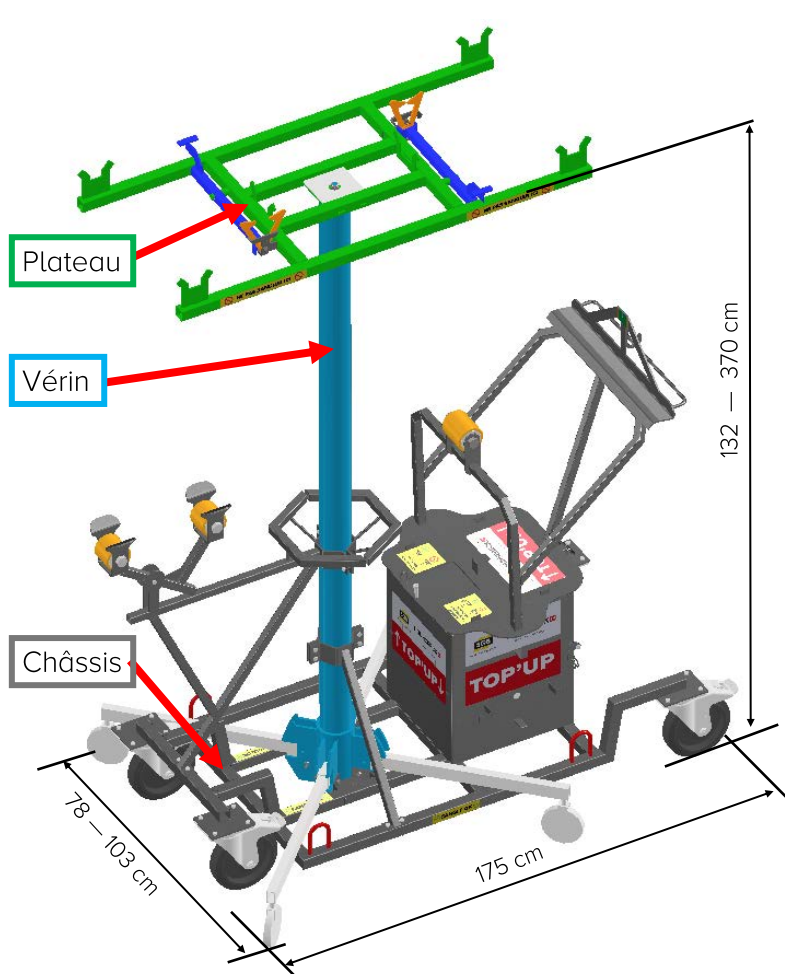
Vue d'ensemble du TOP'UP
